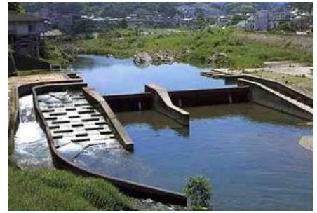
下瀬頭首工
